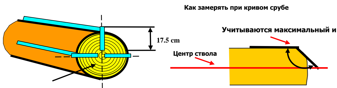
Рис. 35: точки замера угла
