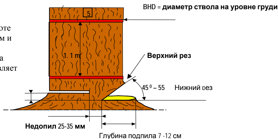
Рис. 9: Измерения и отметки
