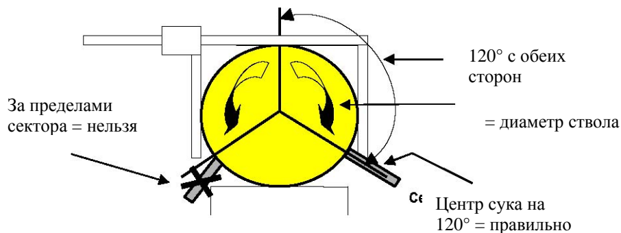
Рис. 38: Область очистки от сучьев слева и справа 120° (соответствует диаметру ствола)
